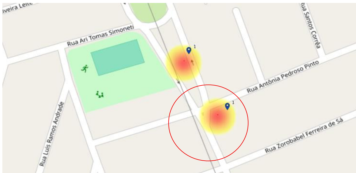
Figura 1. Relatório INFOSIGA.
